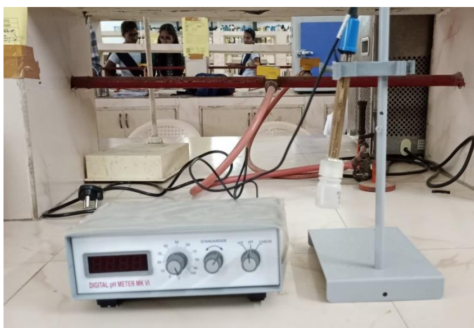
PH METER
